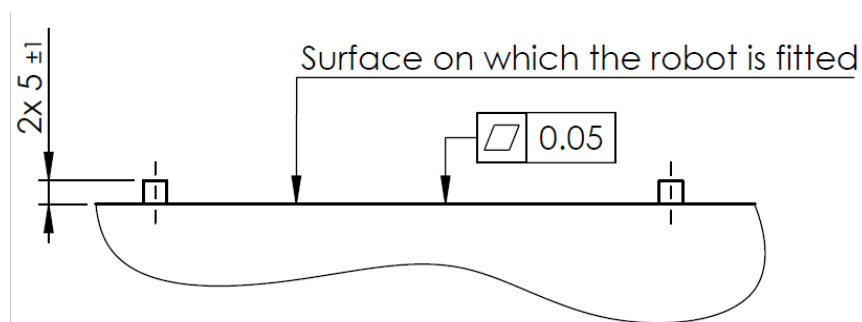
1.2: 機器人底座安裝板
